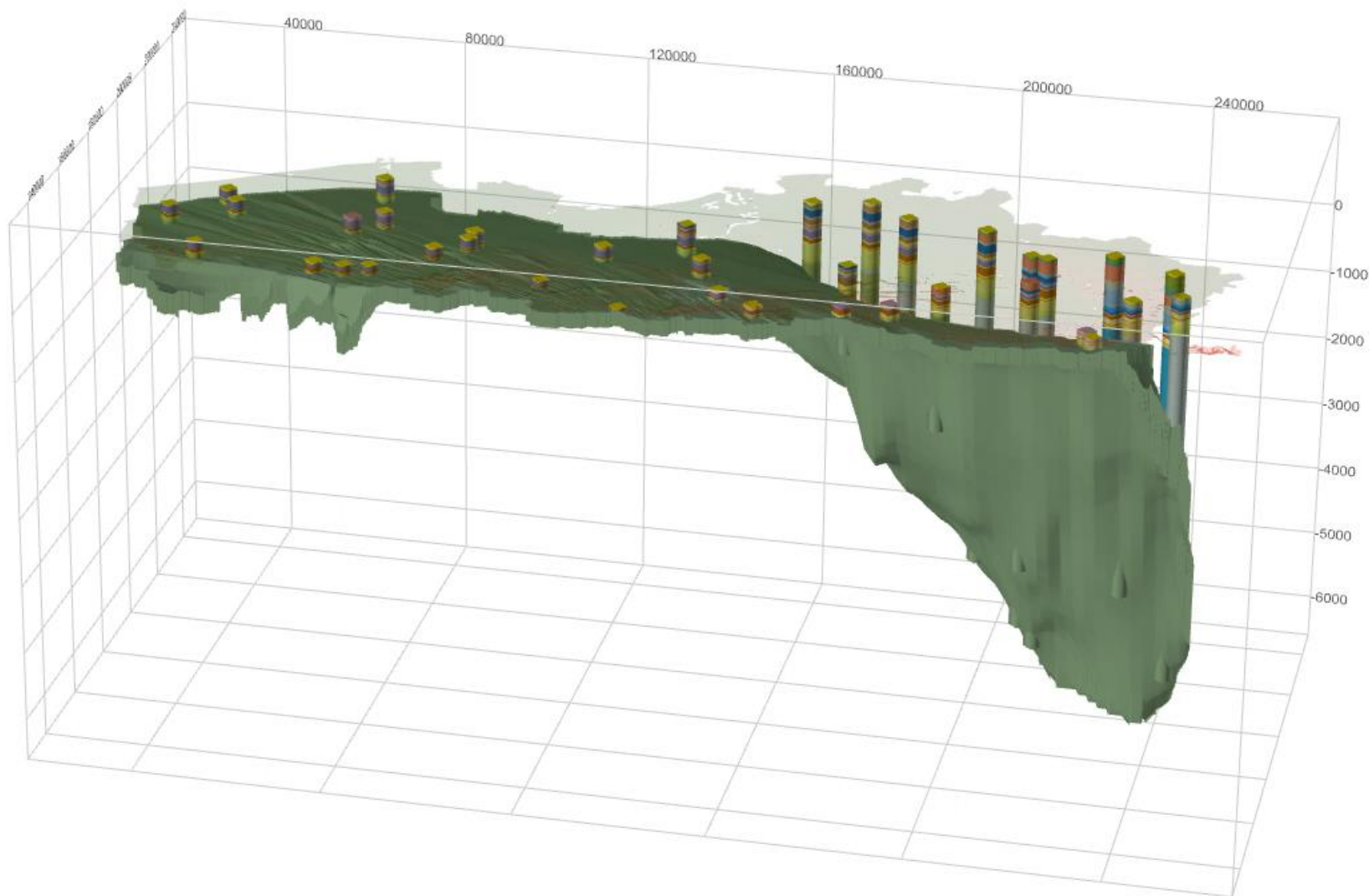
Geologisch 3D Model van Vlaanderen en het Brussels Hoofdstedelijk Gewest, G3Dv2, DOV 2013
